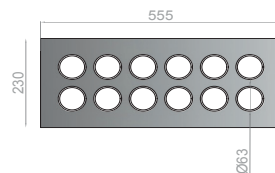
VOORAANZICHT
