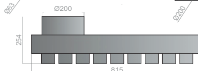
ZIJ-AANZICHT
