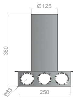
VOORAANZICHT
