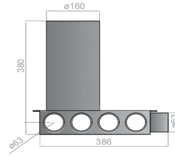
ZIJ-AANZICHT
