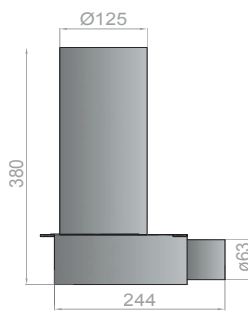
ZIJ-AANZICHT
