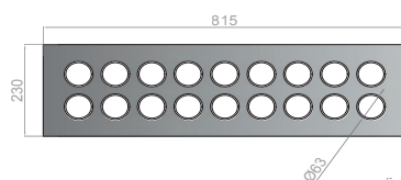
VOORAANZICHT
