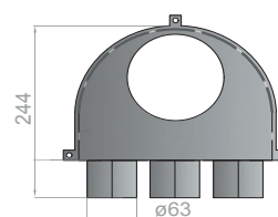
BOVENAANZICHT
