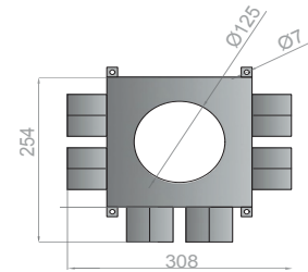
BOVENAANZICHT
