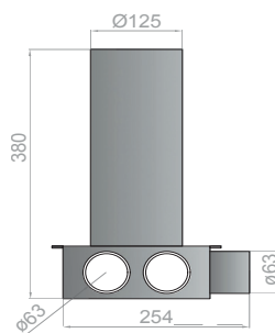
ZIJ-AANZICHT
