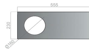
BOVENAANZICHT
