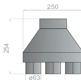
BOVENAANZICHT
