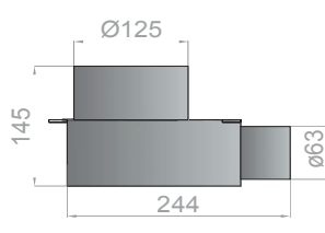
ZIJ-AANZICHT
