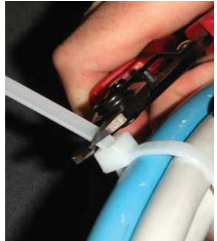
De kabelbinder afknippen op de gewenste lengte met 1 cm veiligheid voor de sterkte.
