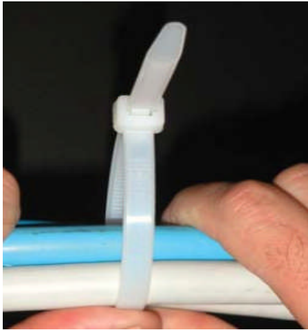
De tip van de kabelbinder door de kop halen.
