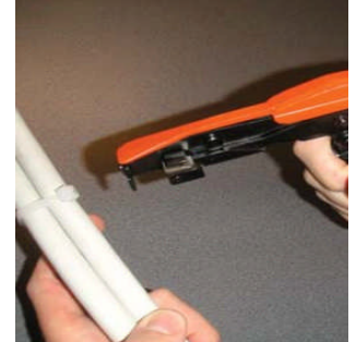
De kabelbinder wordt op de juiste spanning afgeknipt
